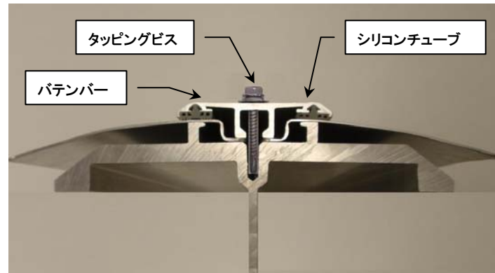
パテン詳細図
