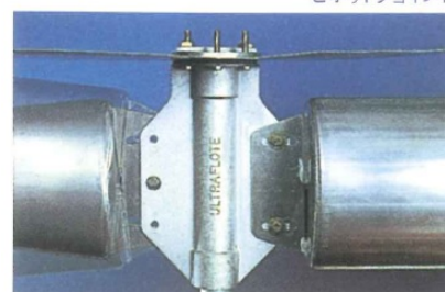
一部分の集中載荷(2,000ポンド以上)に耐える構造 ピボットジョイント
